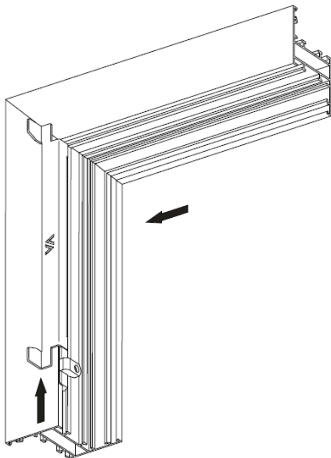
Ribantatre Код 1246.13/.14
