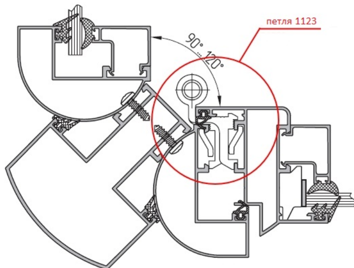
Петля для витражей с поворотом:
